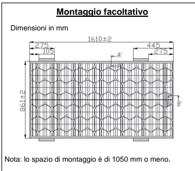
Figura 2-2: Montaggio facoltativo
