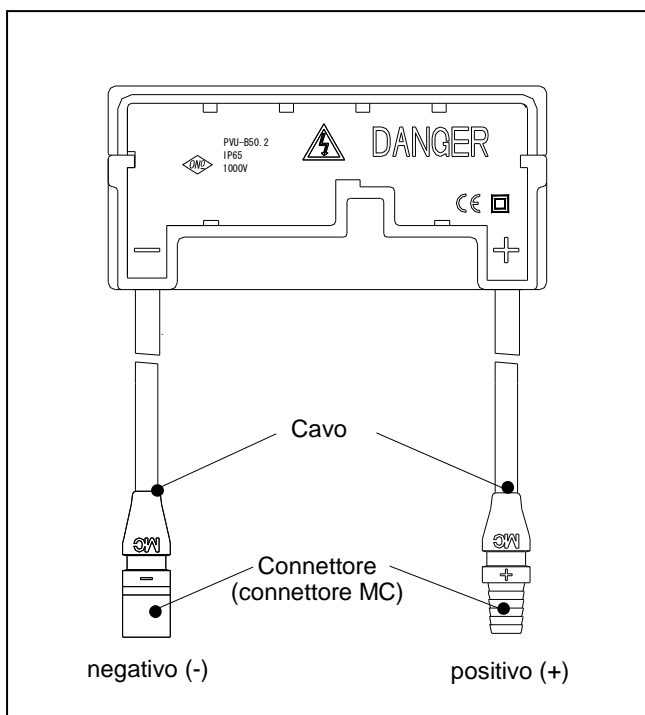
Figura 3: Aspetto della scatola di giunzione
