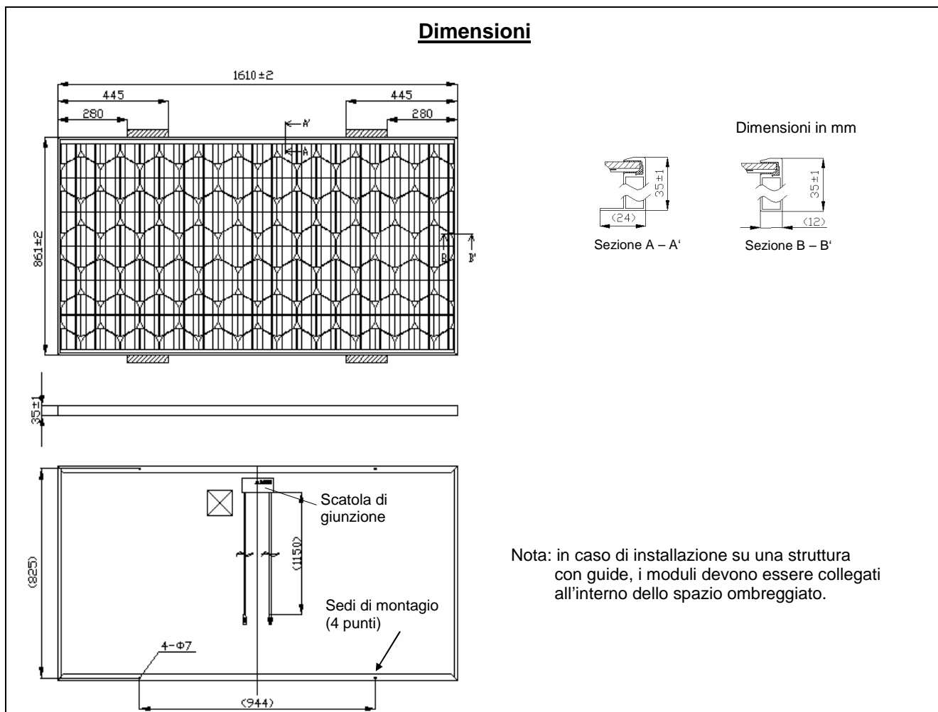
Figura 2-1: Dimensioni
