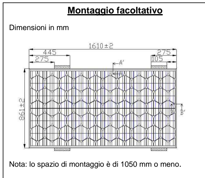
Figura 2-3: Montaggio facoltativo
