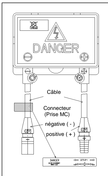
Figure 3: Configuration de la boîte de connexion
