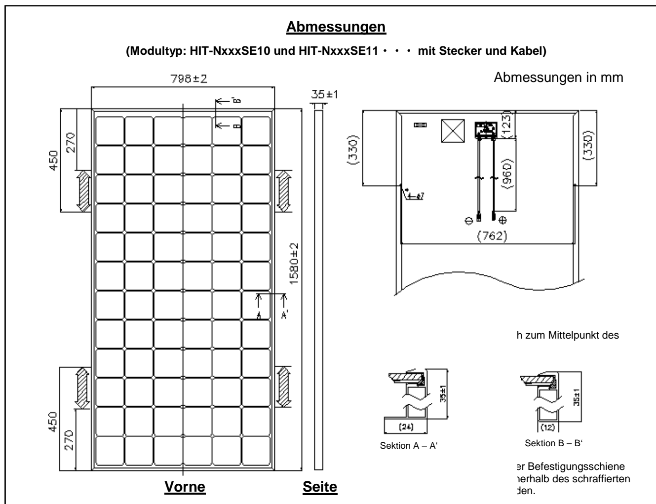
Abb. 2-1: Abmessungen
