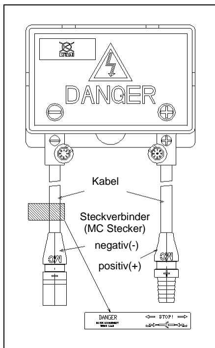
Abb. 2-2: Optionaler Montagebereich
